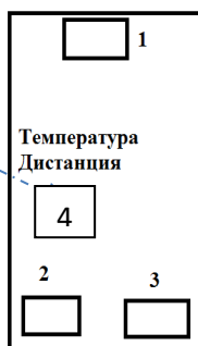
Рис. 4. Схема. Внешний вид монитора «Контроль температуры». 1- Инфракрасный измеритель температуры (погрешность \pm 5\text{ C}^\circ . 2 – кнопка настройки, 3- кнопка меню, 4 - Дисплей NEXTION 480x320 отображает результаты измерения.
